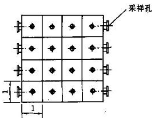
图3 正方形断面的测定点
